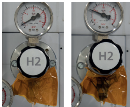
H2 Indikator Tape vor Reaktion
