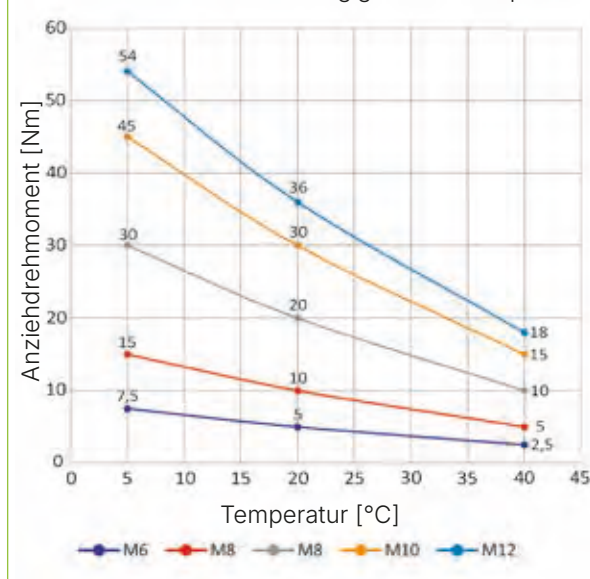
Anziehdrehmoment in Abhängigkeit der Temperatur
