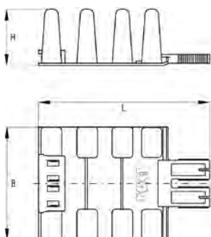
Gleitkufe Typ A
