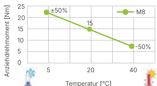
Beispiel Anziehdrehmoment in Abhängigkeit der Temperatur
