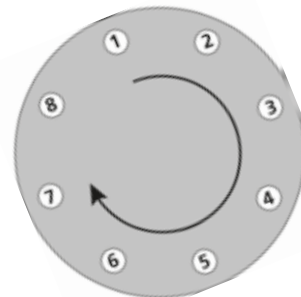
RSG-TW-V (Anzug Schraube)
