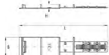
Gleitkufe Typ C
