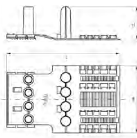
Gleitkufe Typ N
