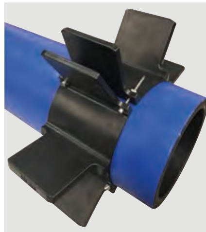
Fertig montierte Gleitkufe
