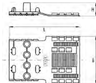
Gleitkufe Typ G
