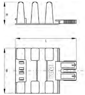
Gleitkufe Typ B
