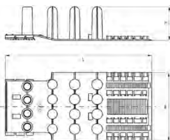
Gleitkufe Typ M
