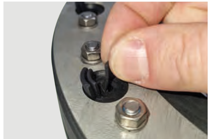
Pressio®-Rings 2 × 40 mm Gumm mit 4 × 6-16 mm Bohrung inkl. Einsatz und Blindstopfen
