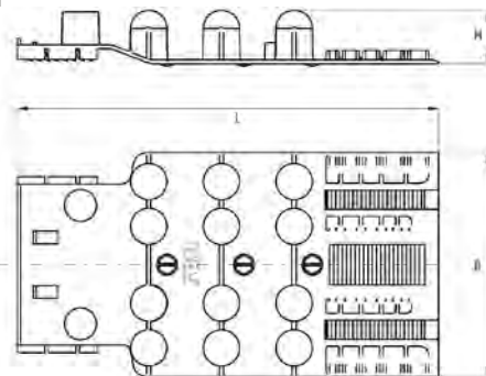
Gleitkufe Typ I
