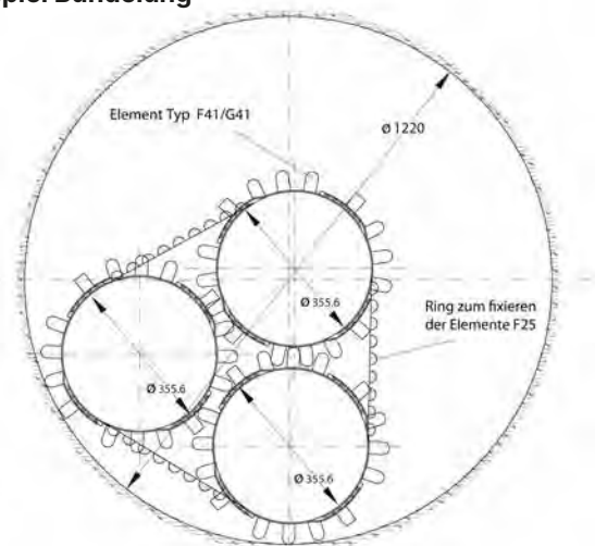
Beispiel Zusatzrohre
